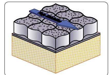
Figura 4. Efecto de la geocelda CONFICELL LS sobre el material de protección.
