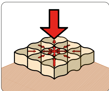
Figura 1. Efecto de confinamiento que aumenta el módulo mecánico de la capa.
